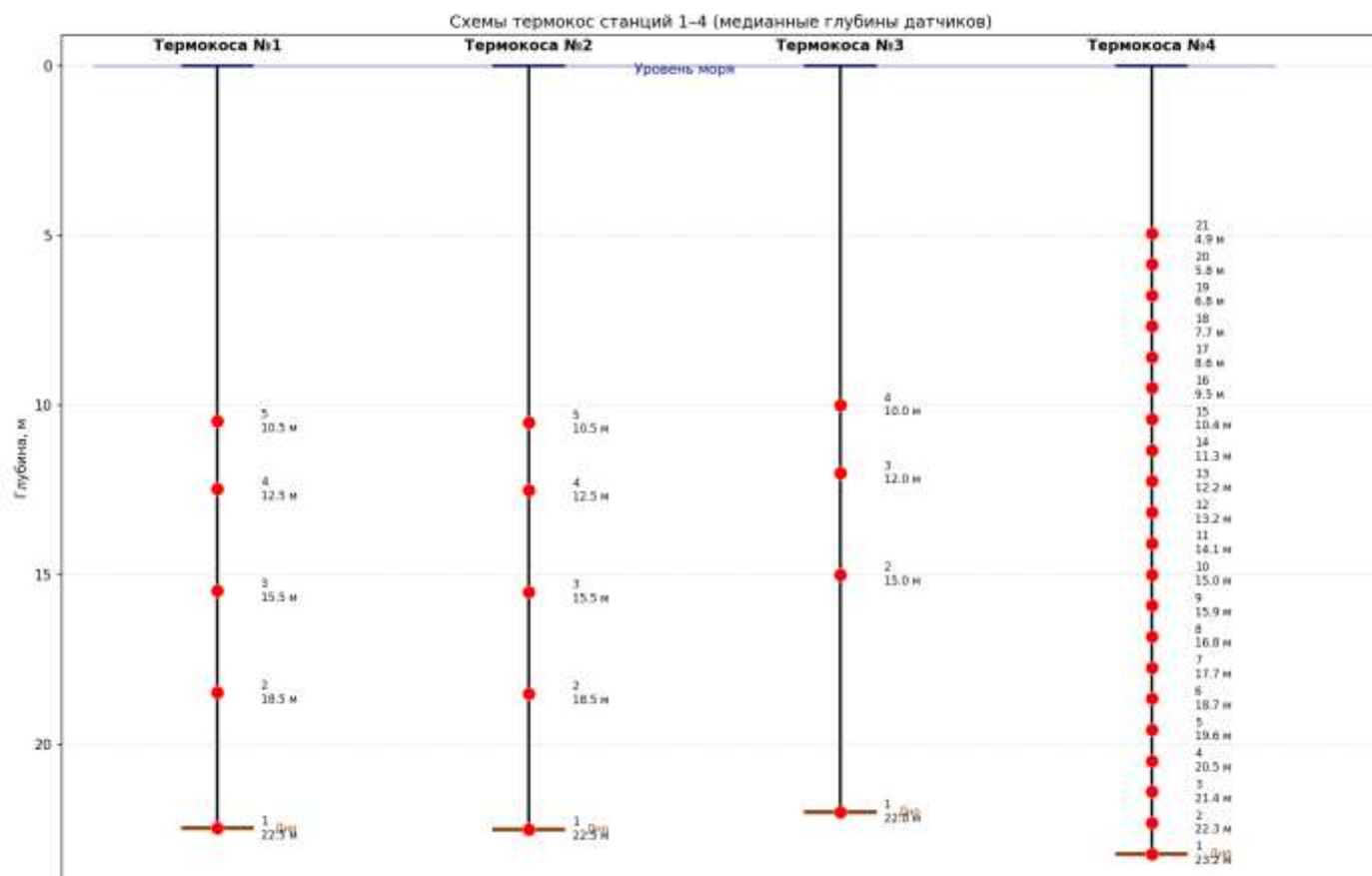
Рис. 4 – Схема термокосы Т1-Т4 с отмеченными датчиками (красный) и их медианными глубинами.
