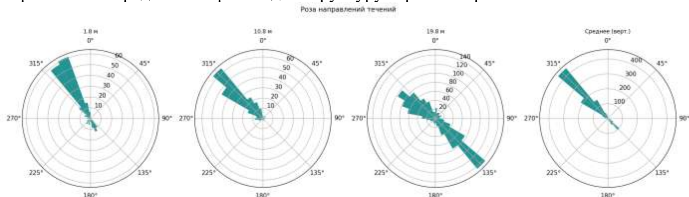
Рис. 15 – Роза направлений течений для тех же горизонтов. Ноль – север, углы по часовой стрелке.
