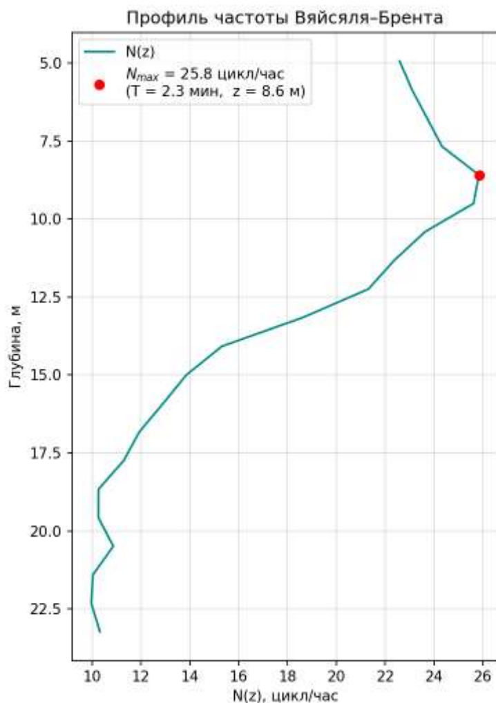
Рис. 2. – Профиль частоты Вяйсяля–Брента с указанным максимальным значением 25.8 цикл/час, период T=2.3 мин.
