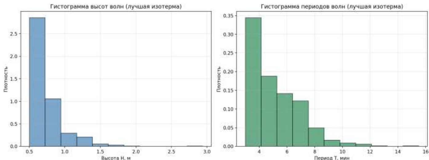
Рис. 19 – Распределение параметров короткопериодных внутренних волн на изотерме 15,5 °С: а – гистограмма высот волн H (м); б – гистограмма периодов волн T (мин).
