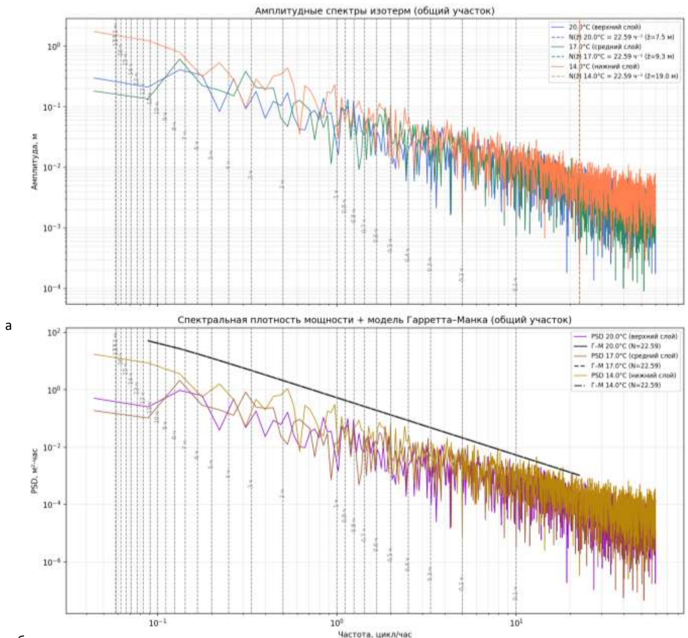
Рис. 10 – Результаты спектрального анализа вертикальных смещений изотерм на общем непрерывном участке (22,6 ч): а – амплитудные спектры (FFT) для изотерм 14, 17 и 20 °С; б – спектральная плотность мощности (PSD) для тех же изотерм (цветные линии) и модель Гарретта–Манка (чёрные линии разного стиля). Вертикальная пунктирная линия соответствует частоте Вайсяля–Брента N \approx 22,6 \text{ ч}^{-1} .
