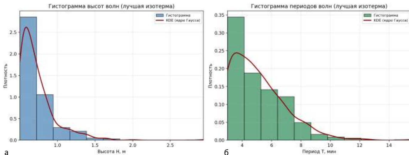
Рис. 20 – Распределения высоты ( H ) и периода ( T ) волн на лучшей изотерме 15.5 °C (непрерывный участок записи): гистограммы и сглаженные оценки плотности (KDE, гауссово ядро).
