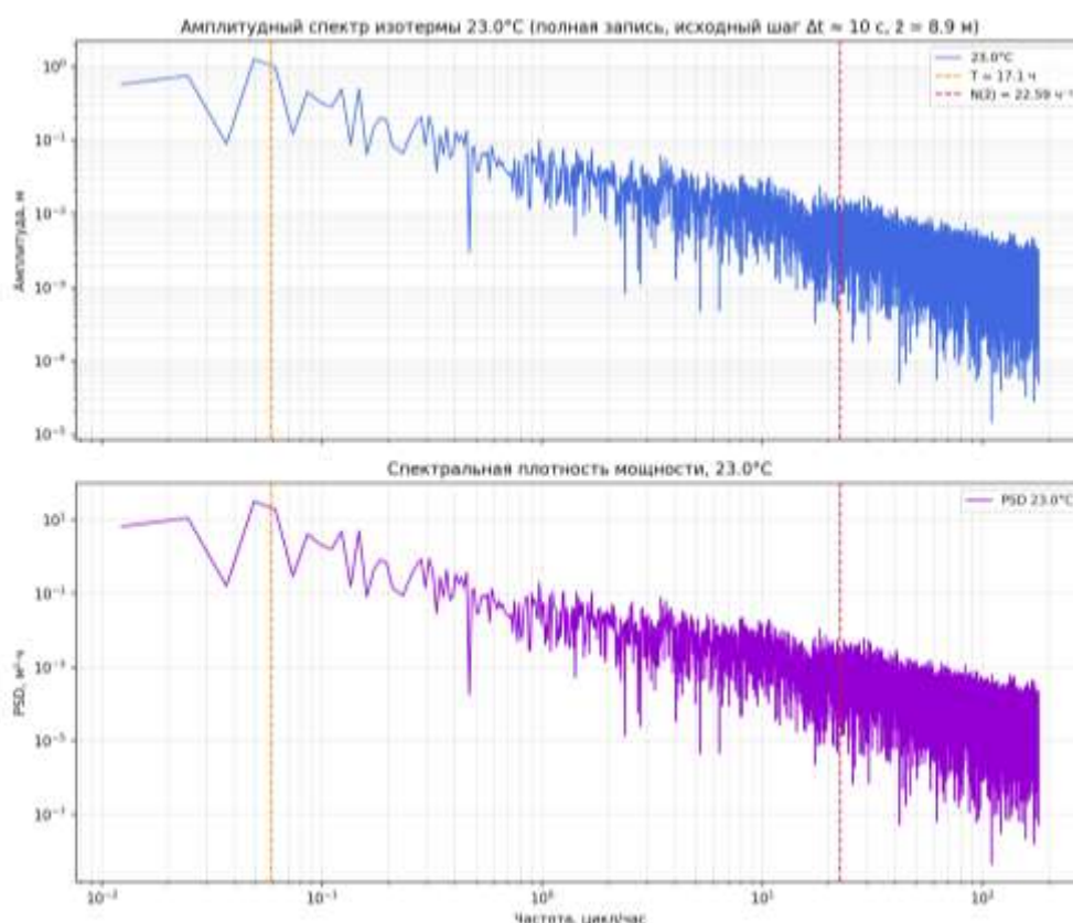
Рис. 9 – Амплитудный спектр (а), спектральная плотность мощности (б) изотермы 23°C с пиком на частоте 17.1ч
