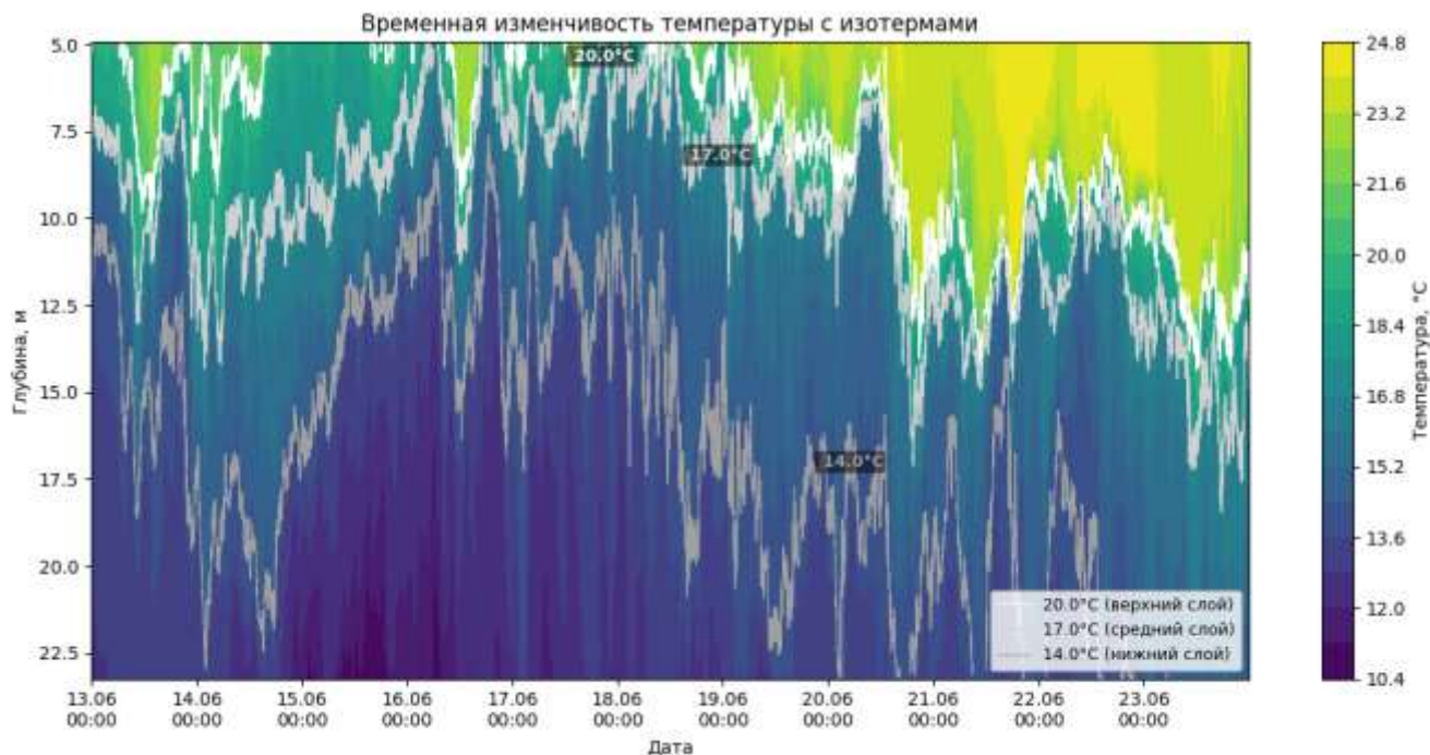
Рис. 7 – Временные колебания изотерм 14°C, 17°C, 20°C.
