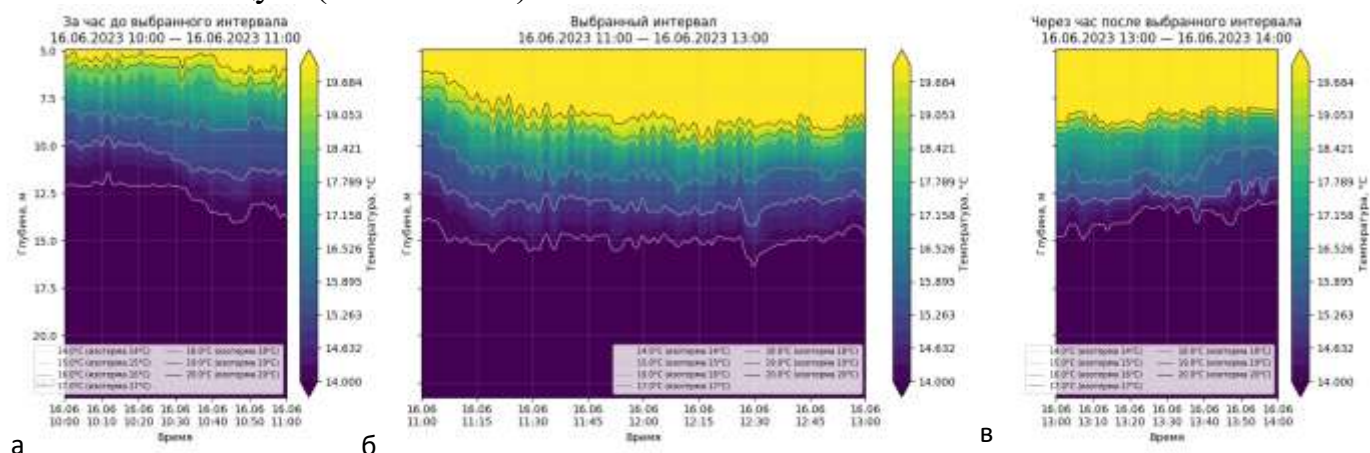
Рис. 22 – Вертикальные смещения изотерм в диапазоне 14–20 °С в окрестности цуга 16.06.2023: (а) – час до цуга (10:00–11:00), (б) – цуг короткопериодных внутренних волн (11:00–13:00), (в) – час после цуга (13:00–14:00). Цветовая шкала соответствует температуре воды, °С.
