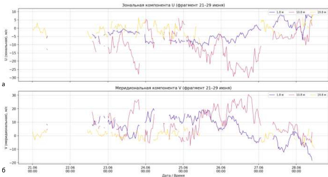
Рис. 13 – Временные ряды компонент скорости U (а) и V(б) на горизонтах 1.8 и 10.8 м в период 21–29 июня 2023 г.
