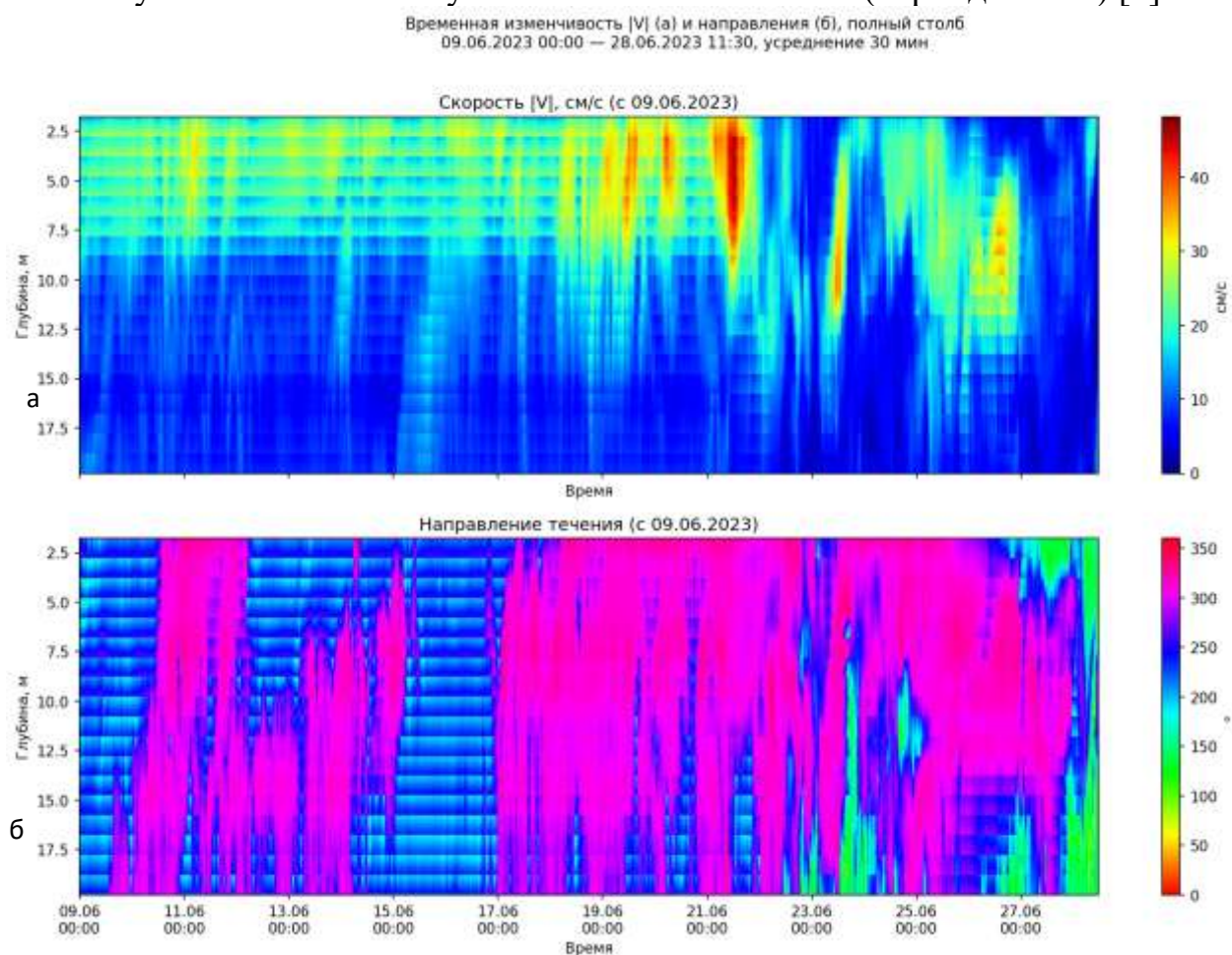
Рис. 11 – Временная изменчивость скорости течения |V| (а) и его направления (б) по данным ADCP (усреднение 30 мин).
