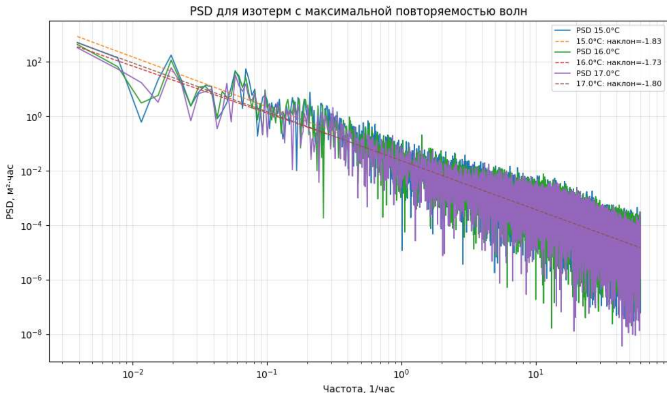
Рис. 21 – Спектральная плотность мощности (PSD) для изотерм 15,0; 16,0; 17,0 °С (наибольшая повторяемость волн). Пунктирными линиями показаны линейные аппроксимации наклона.
