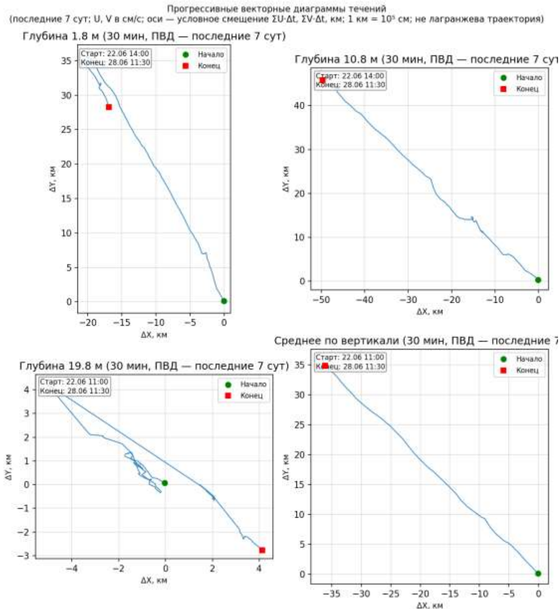
Рис. 17 – Прогрессивные векторные диаграммы течений ( X = \Sigma U \cdot \Delta t, Y = \Sigma V \cdot \Delta t ) для горизонтов 1,8; 10,8; 19,8 м и вертикального среднего. Начало – зелёный маркер, конец – красный.
