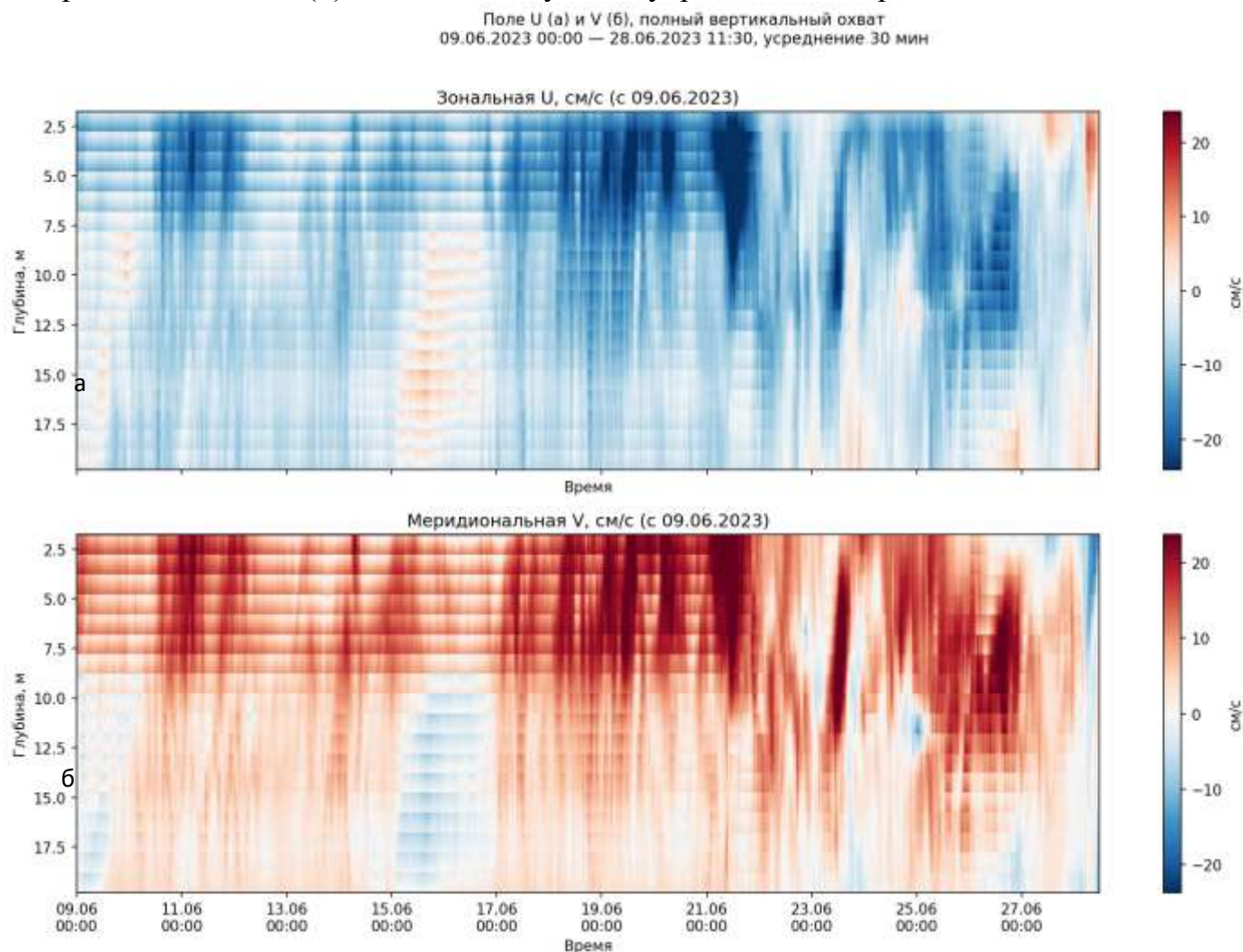
Рис. 12 – Поле временной изменчивости для зональной компоненты U (а) и меридиональной V (б). Усреднение 30 мин, красный – положительные значения (восток/север), синий – отрицательные (запад/юг).
