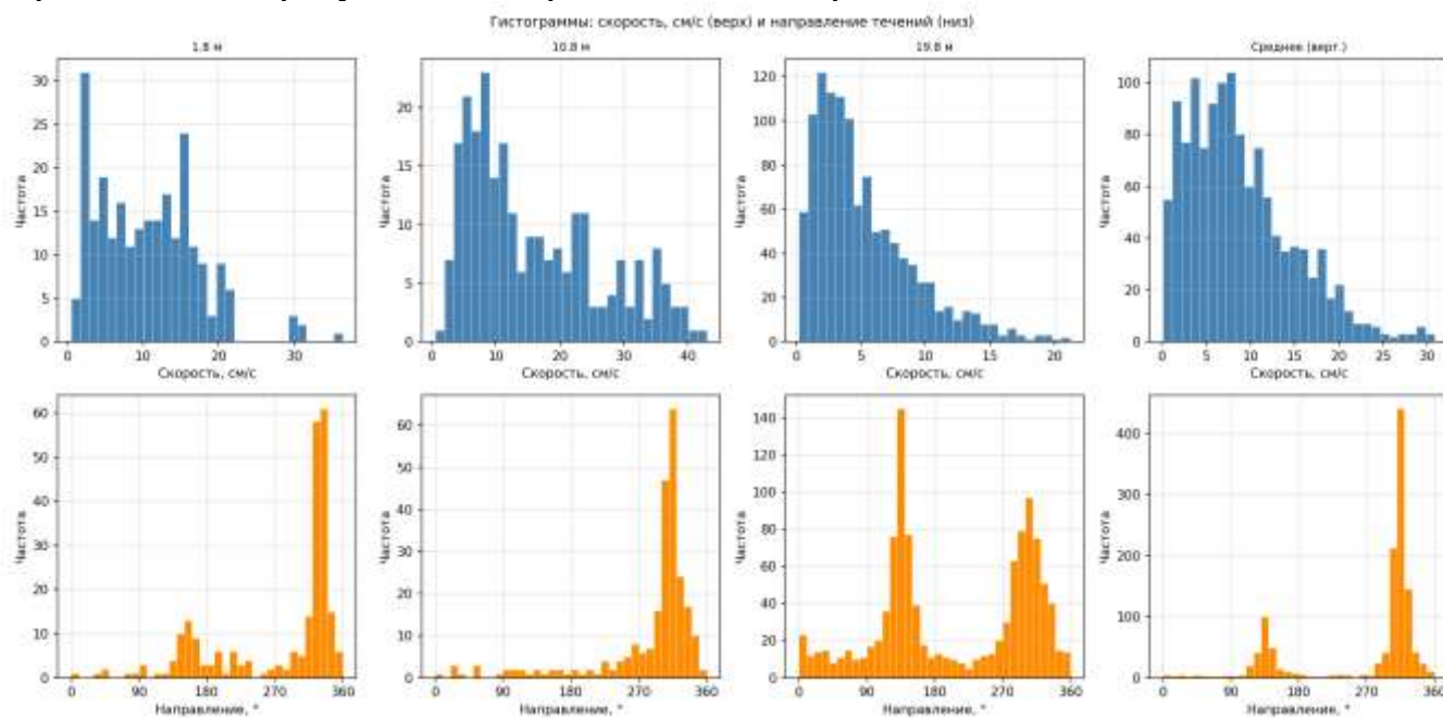
Рис. 14 – Гистограммы скорости (верх) и направления (низ) течений для горизонтов 1,8; 10,8; 19,8 м и вертикального среднего.
